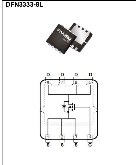
DFN3333-8L
