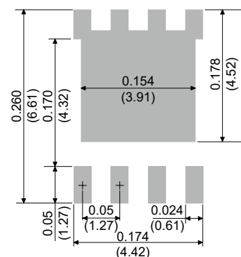
DFN5060-8L
