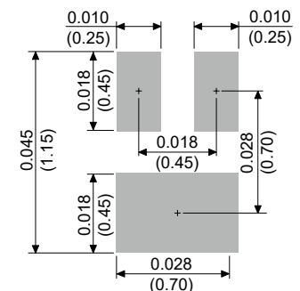
DFN1006T-3L
