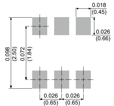
SOT-363
