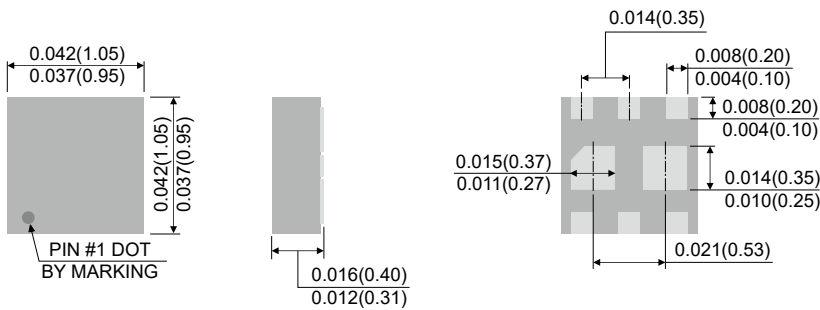
DFN1010B-6L
