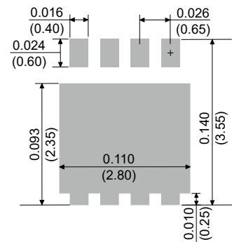
DFN3333B-8L
