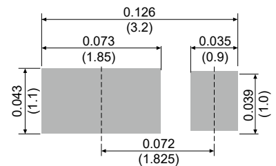
SOD-323HE
