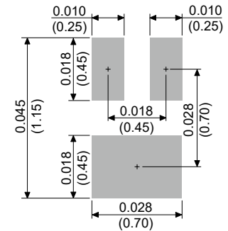
DFN1006T-3L
