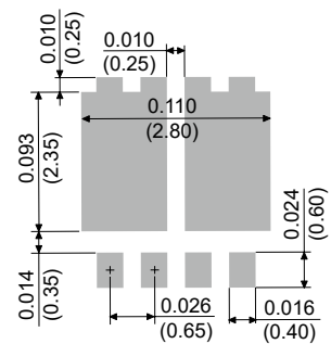
DFN3333B-8L
