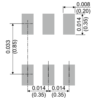
DFN1010B-6L
