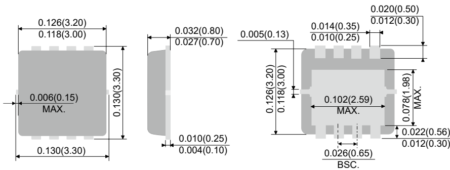
DFN3333-8L
