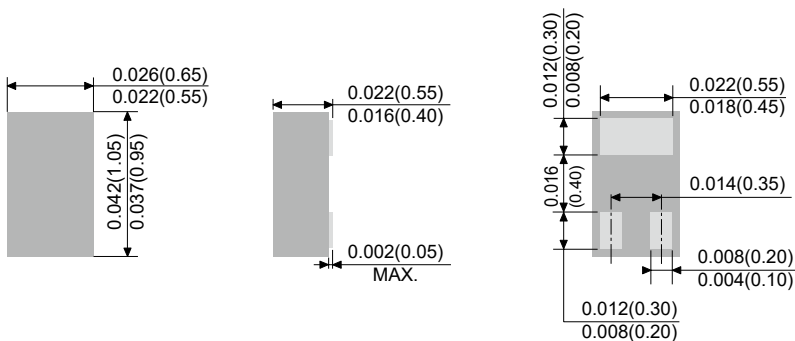
DFN1006T-3L
