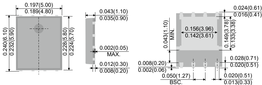
DFN5060-8L
