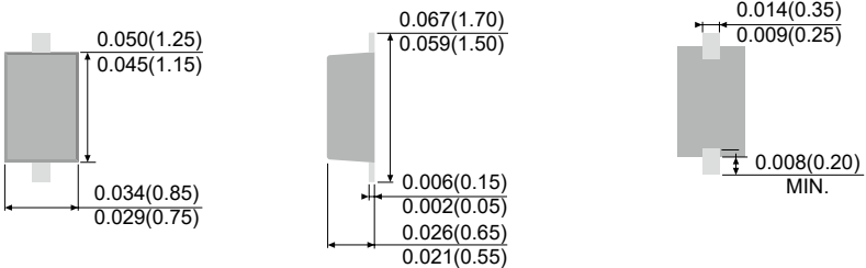
SOD-323HE
